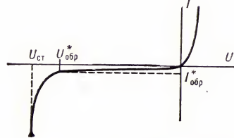
Рис. 2. Типичная вольт-амперная характеристика полупроводникового диода с p-n -переходом: U — напряжение на диоде; I — ток через диод; U^*_{обр} и I^*_{обр} — максимальное допустимое обратное напряжение и соответствующий обратный ток; U_{ст} — напряжение стабилизации.
